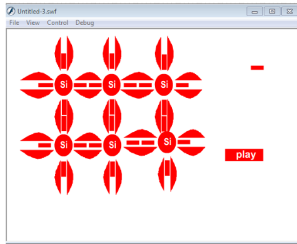
Gambar 2. Electron valensi
